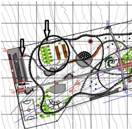
Εικόνα 2: Θέση των δύο υφιστάμενων βλαφθέντων κτηρίων προς επισκευή και η θέση προτεινόμενων μεταλλικών στεγάστρων.
